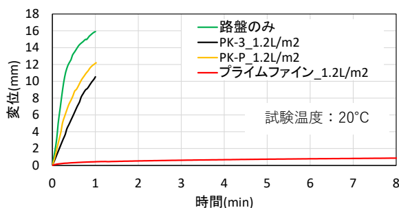
ホイールトラッキング試験による変形抵抗性能
